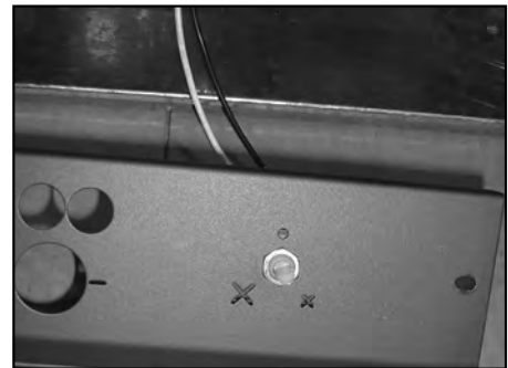
Figure 44. Install Fan Control Nut.
