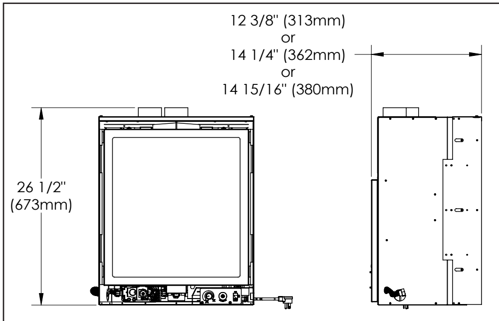
Figure 37: Q1 Insert Dimensions
