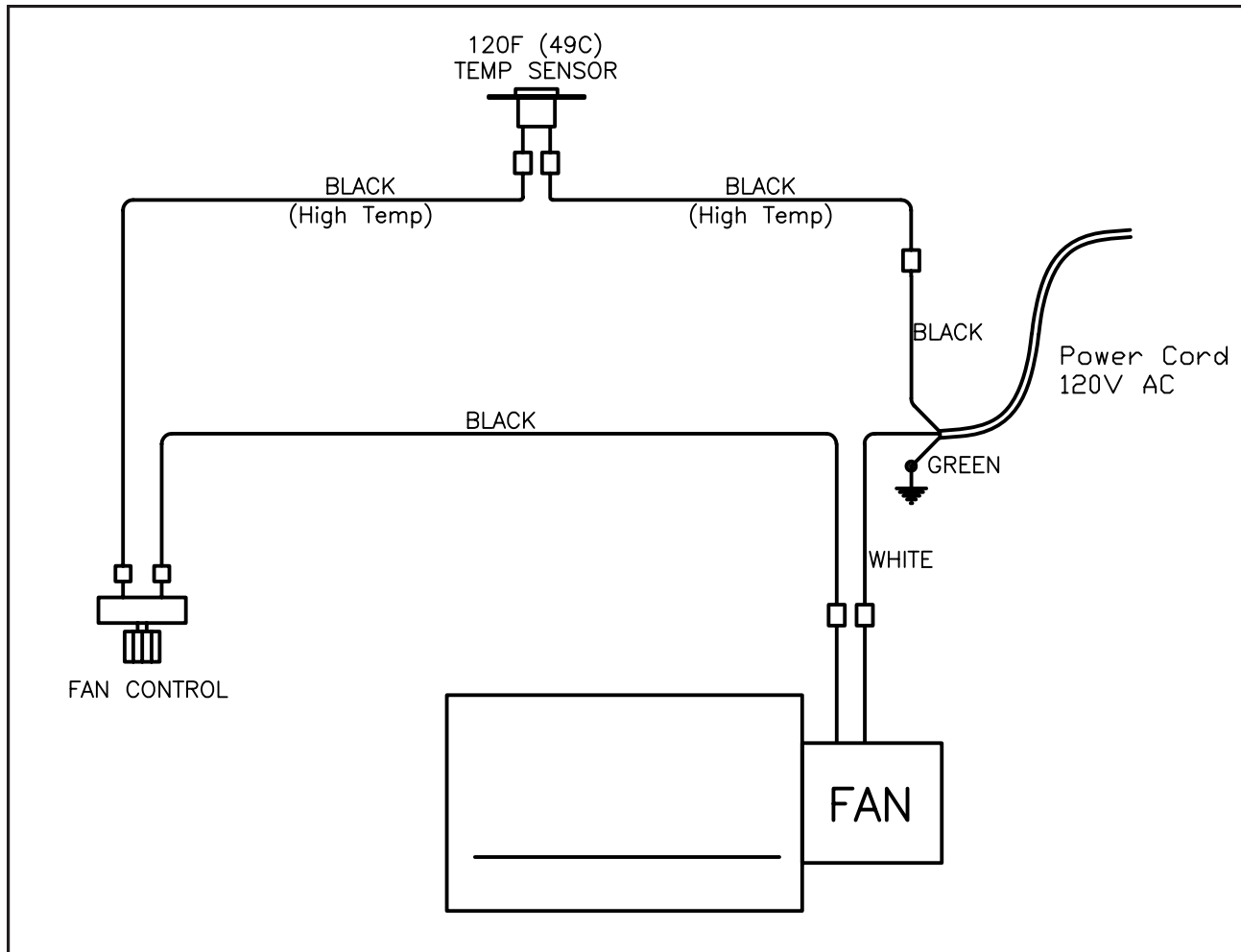
Figure 50: Fan wiring diagram.
